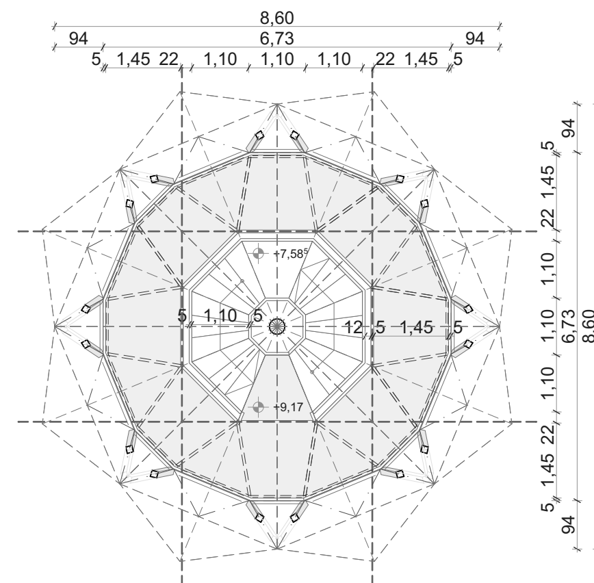
2. kilátószinti alaprajz (+9,17m):
