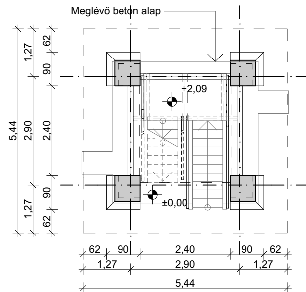
Földszinti alaprajz (+0,00m):
