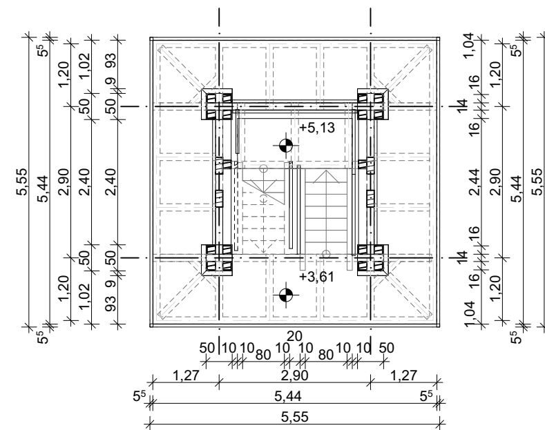
1. kilátószinti alaprajz (+3,61m):
