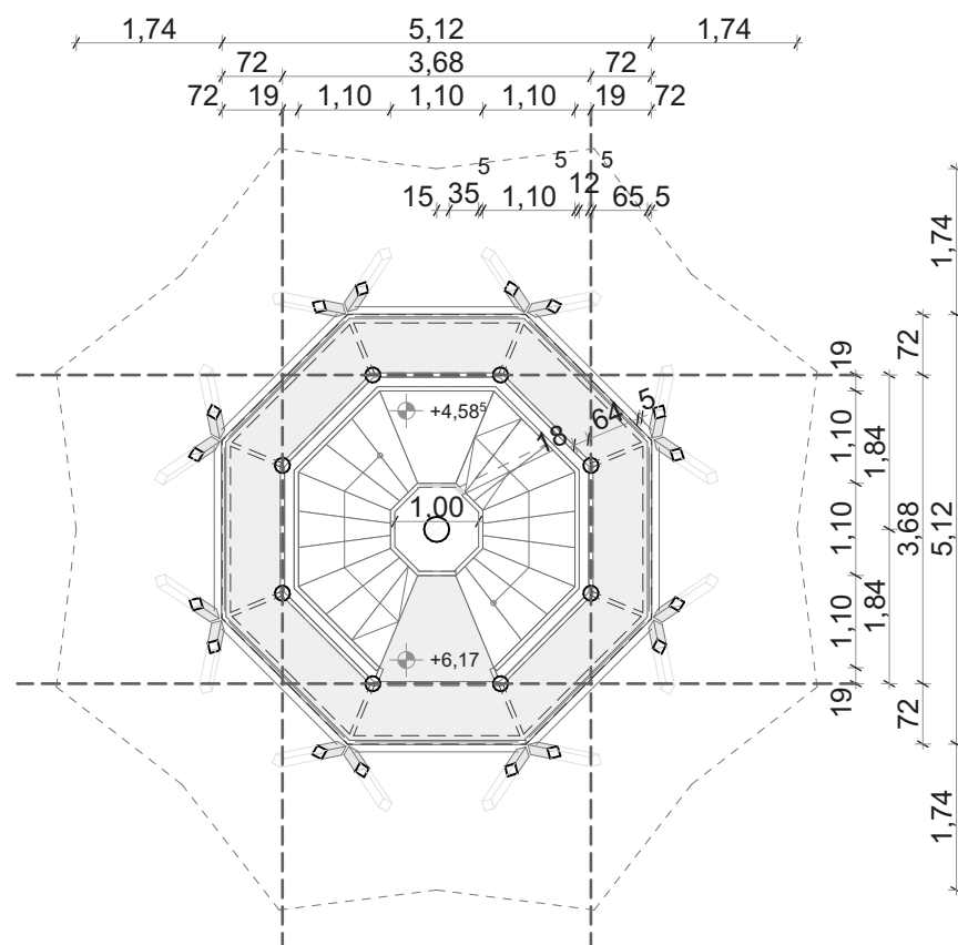
1. kilátószinti alaprajz (+6,17m):
