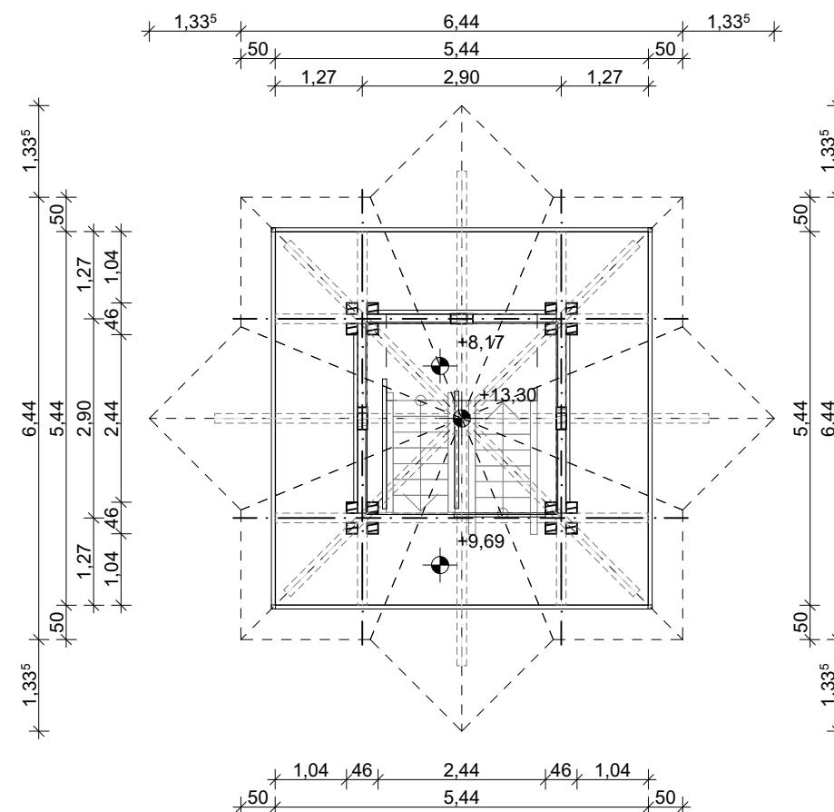
3. kilátószinti alaprajz (+9,69m):
