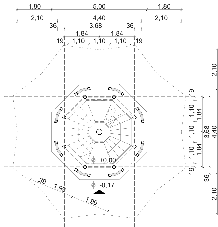
Földszinti alaprajz (+0,00m):
