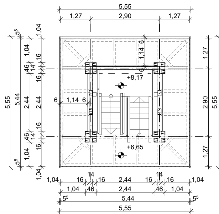
2. kilátószinti alaprajz (+6,65m):
